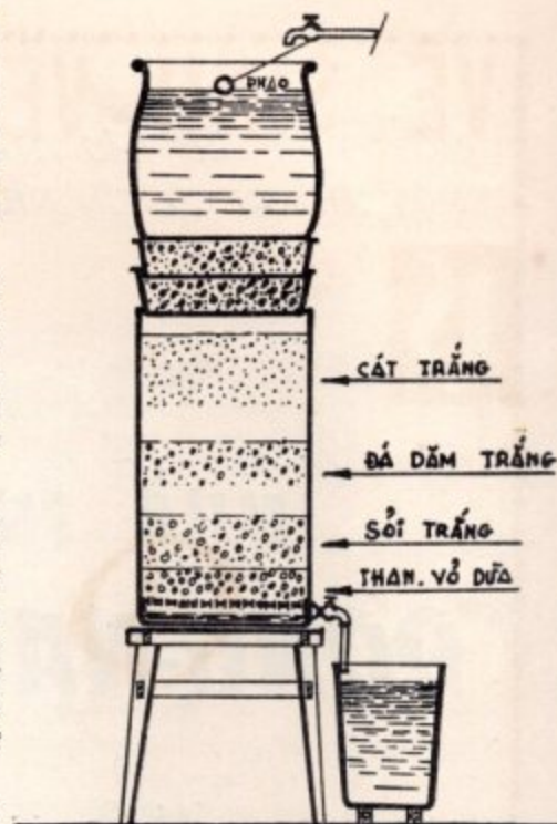
Giản Đồ Máy Lọc Nước
