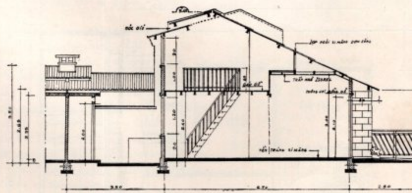
THIẾT ĐỒ (có gác)
