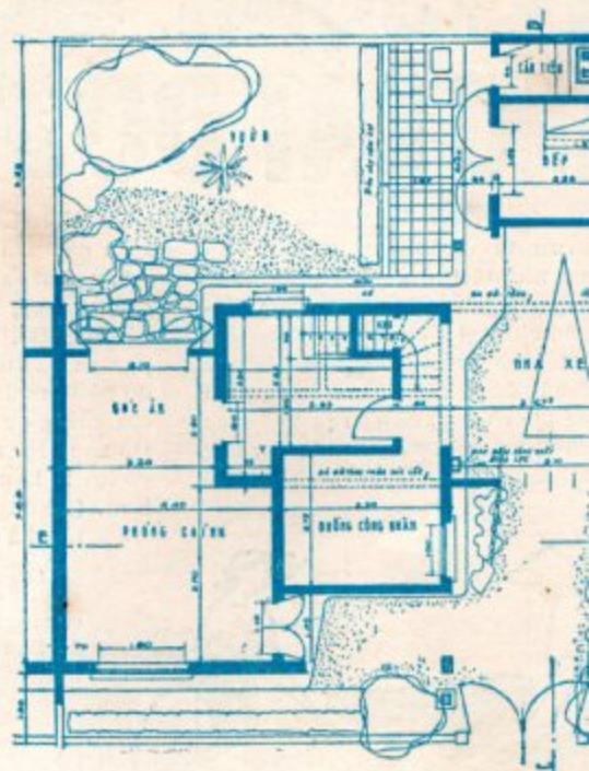
BÌNH ĐỒ NHÀ DƯỚI
