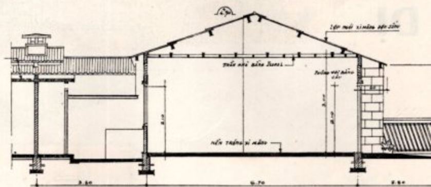
THIẾT ĐỒ (không có gác)
