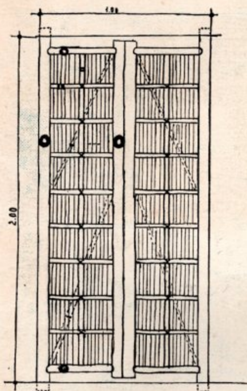
MỘT CÁI CỬA RA VÀO 2 CẠNH TOÀN ĐẲNG TRE. CẠNH CỬA ĐÓNG TRE HAI CÁI CỐI GỖ CÙNG KIỂU C
