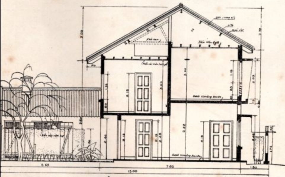
XẼ ĐỌC THEO A-B
