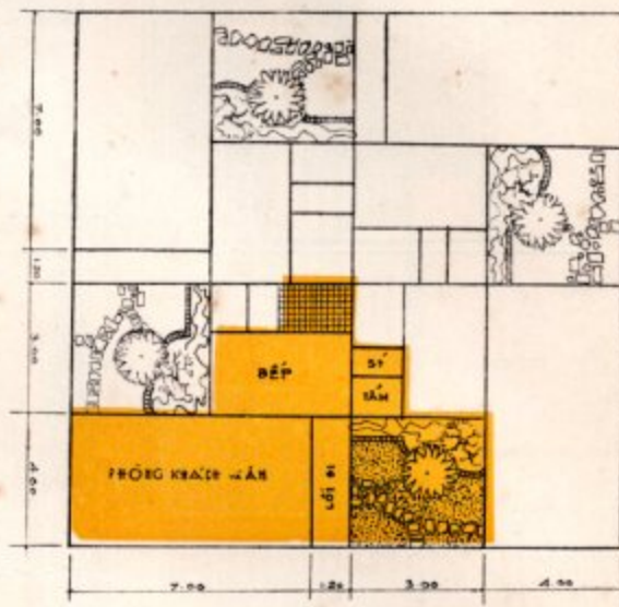
BÌNH ĐỒ 'TỨ' LẬP
