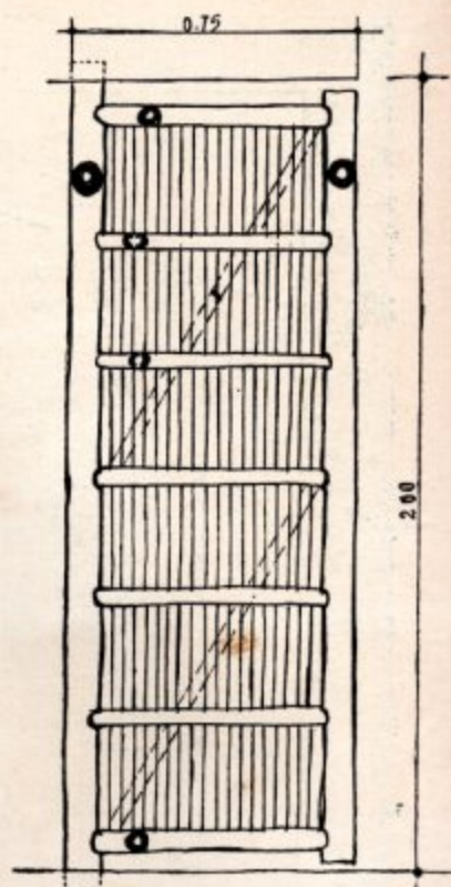
PHÉP CHÉ CỦA SỖ ĐẲNG NỨA MỘC CÁP LÊN XƯƠNG
