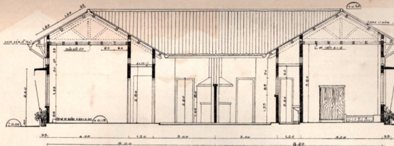
THIẾT ĐỒ
