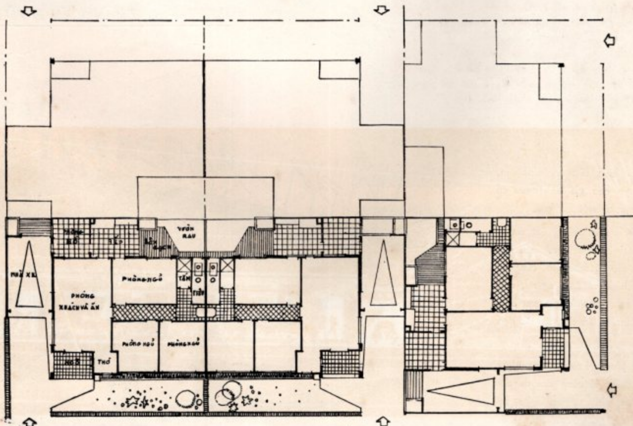
BÌNH ĐỒ
