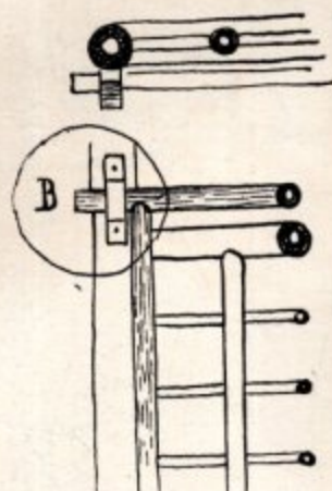
CHÂN ĐÓNG CỦA SỖ ĐẲNG GỖ HAY TRE VỚI CÁC LAO MÀN
