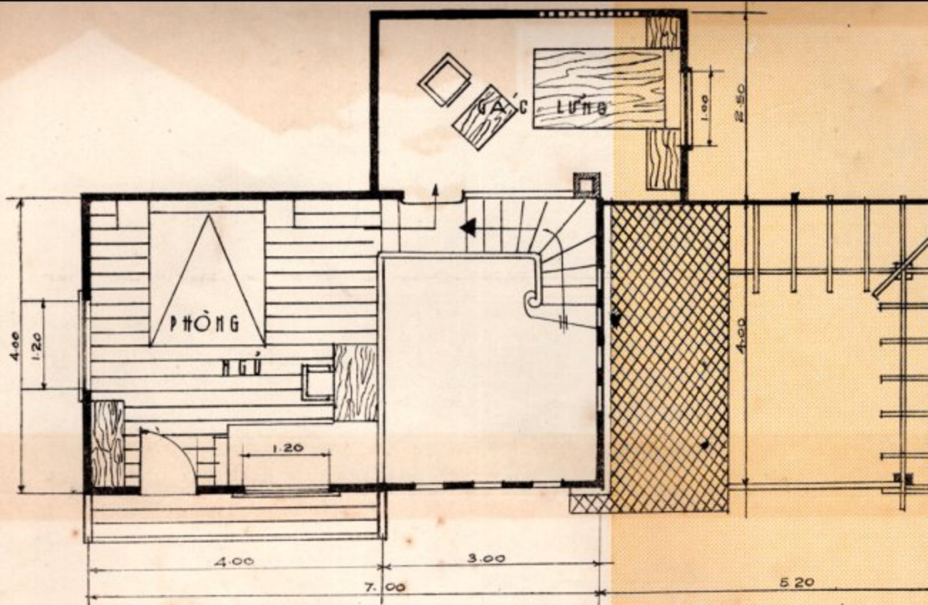
BÌNH ĐỒ TẦNG GÁC
