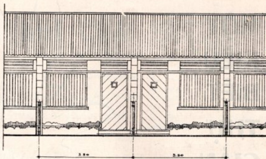
CHÍNH DIỆN (không có gác)
