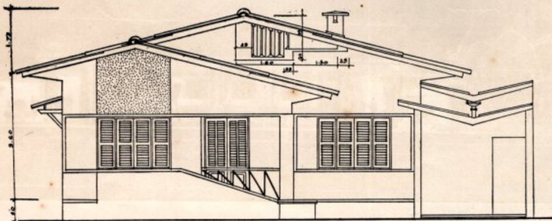
CHÍNH DIỆN
