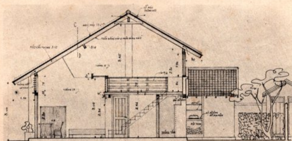
THIẾT ĐỒ ĐỌC THEO AB
