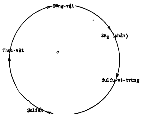
VÒNG TUẦN HOÀN CỦA SULFU
